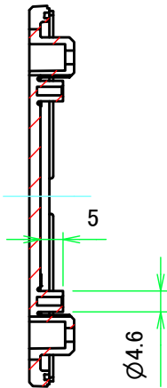
E-E ( 1 : 1.5 )
