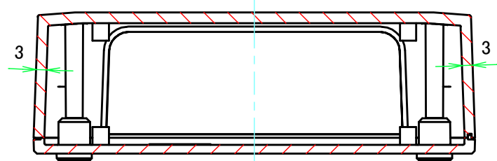
B-B ( 1 : 1.5 )
